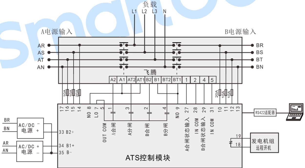
图10 飞腾应用图
