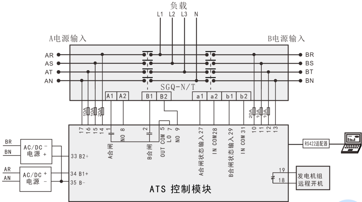
图9 SGQ-N/T 应用图
