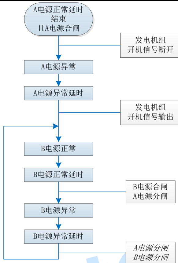
图4 自投不自复(互为备用无效)流程图
