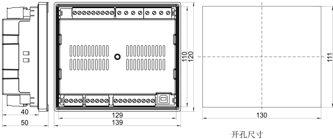
图13 外形尺寸及面板开孔尺寸
