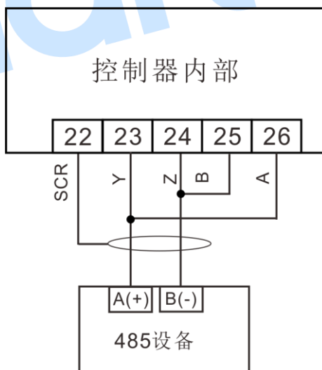
图5 与485设备连接示意图
