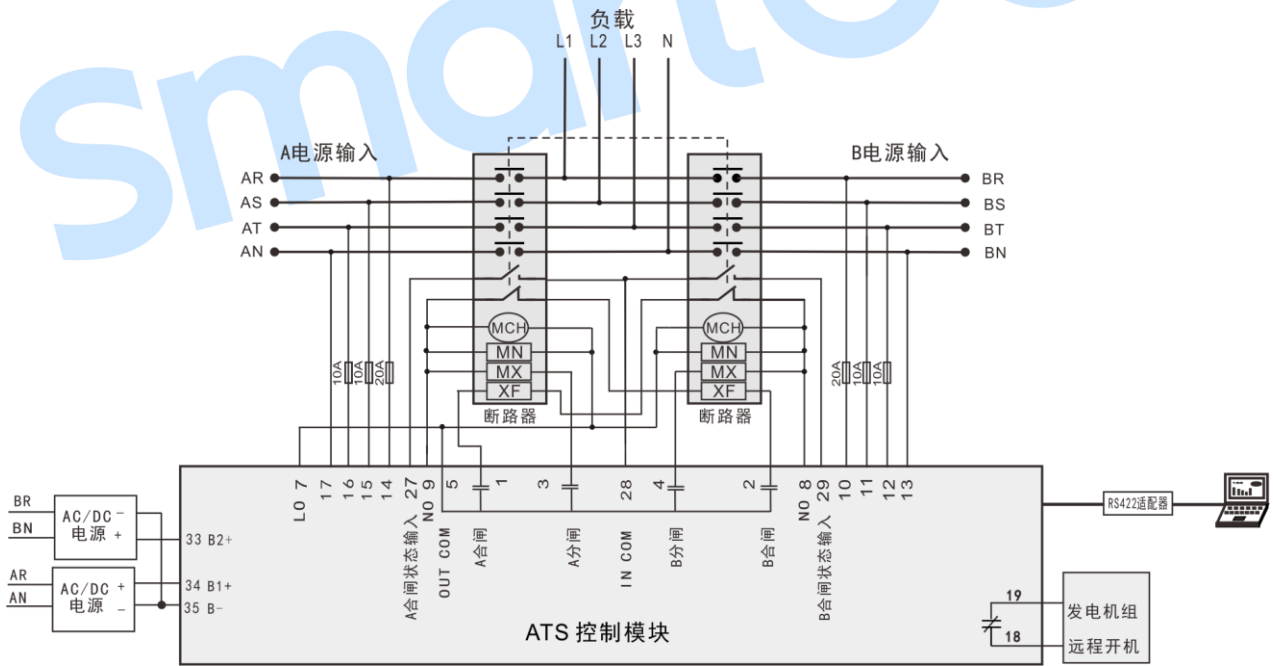
图12 断路器(ACB)应用图
