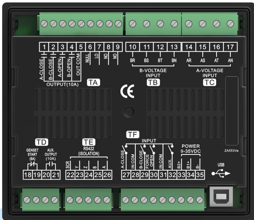
图8 控制器后面板图
