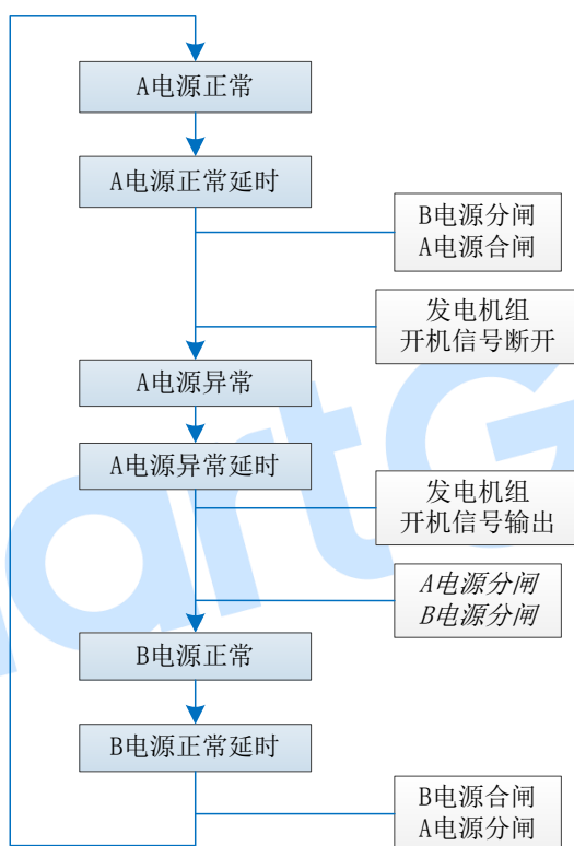
图2 自投自复流程图
