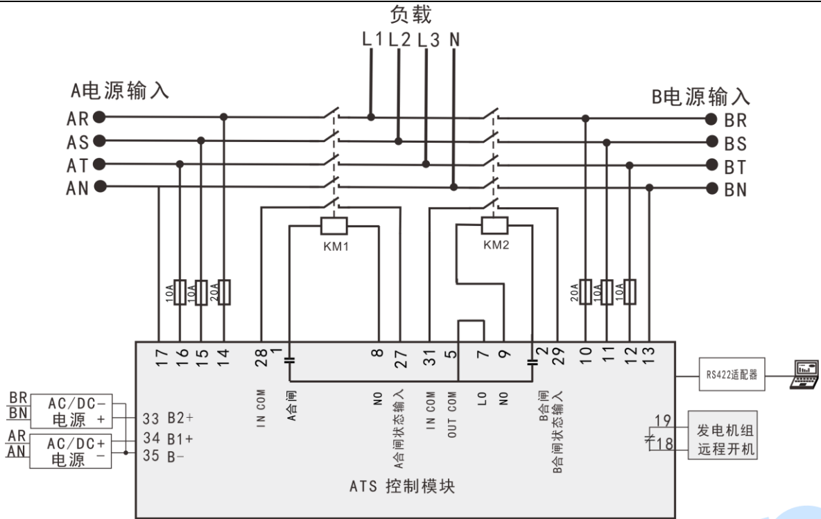
图11 接触器应用图
