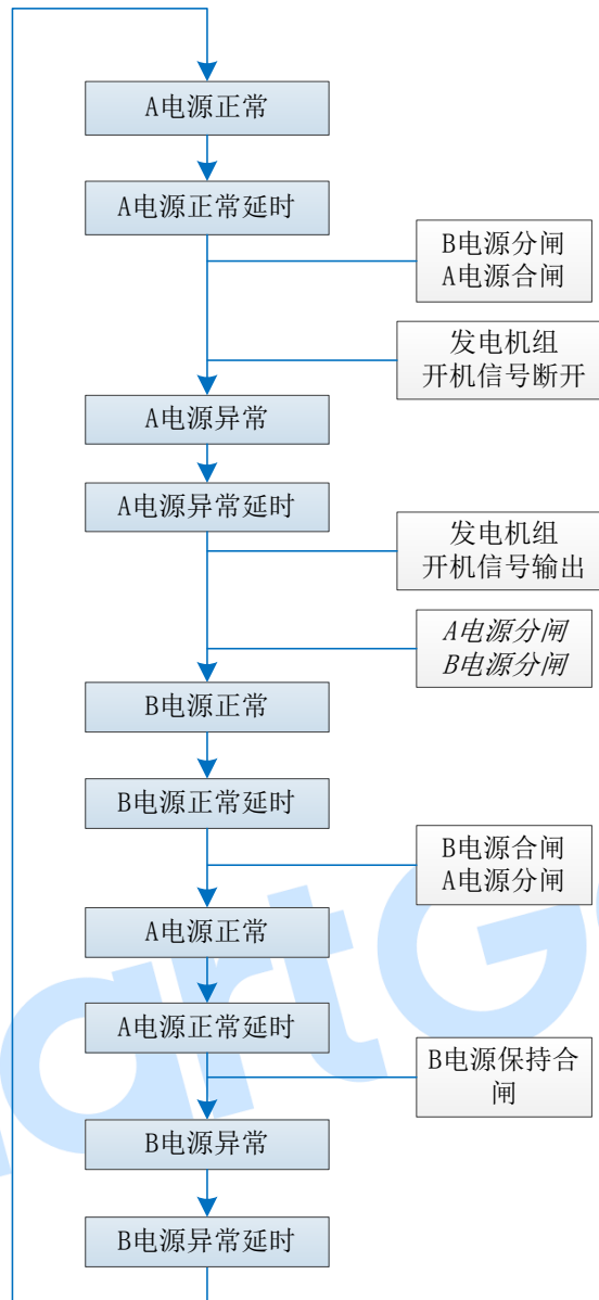
图3 自投不自复(互为备用有效)流程图
