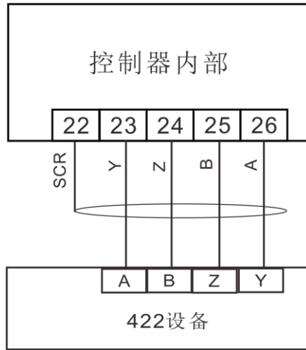
图6 与 422 适配器连接示意图
