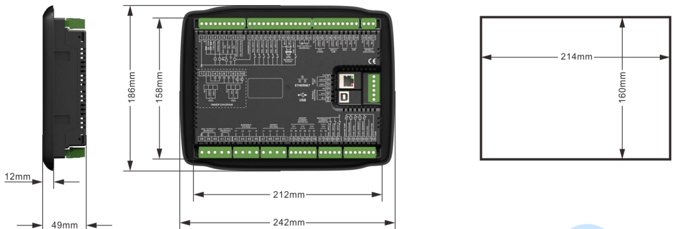
图17 外形尺寸及面板开孔尺寸
