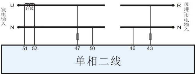
图13 单相二线应用图
