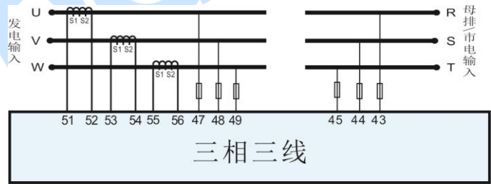
图11 三相三线应用图
