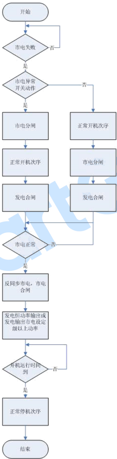
图8 AMF 模式
