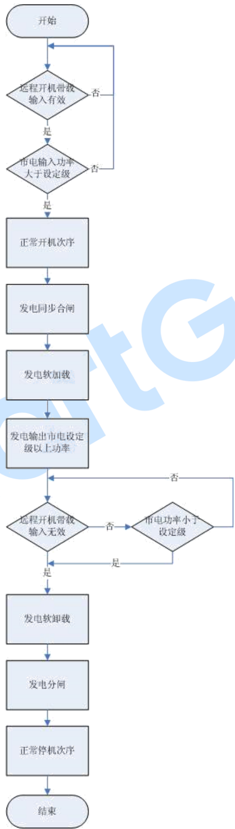
图6 市电剪峰模式
