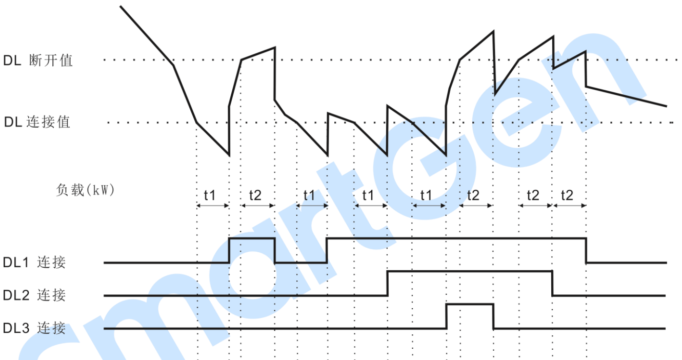
图16 DL 时序
