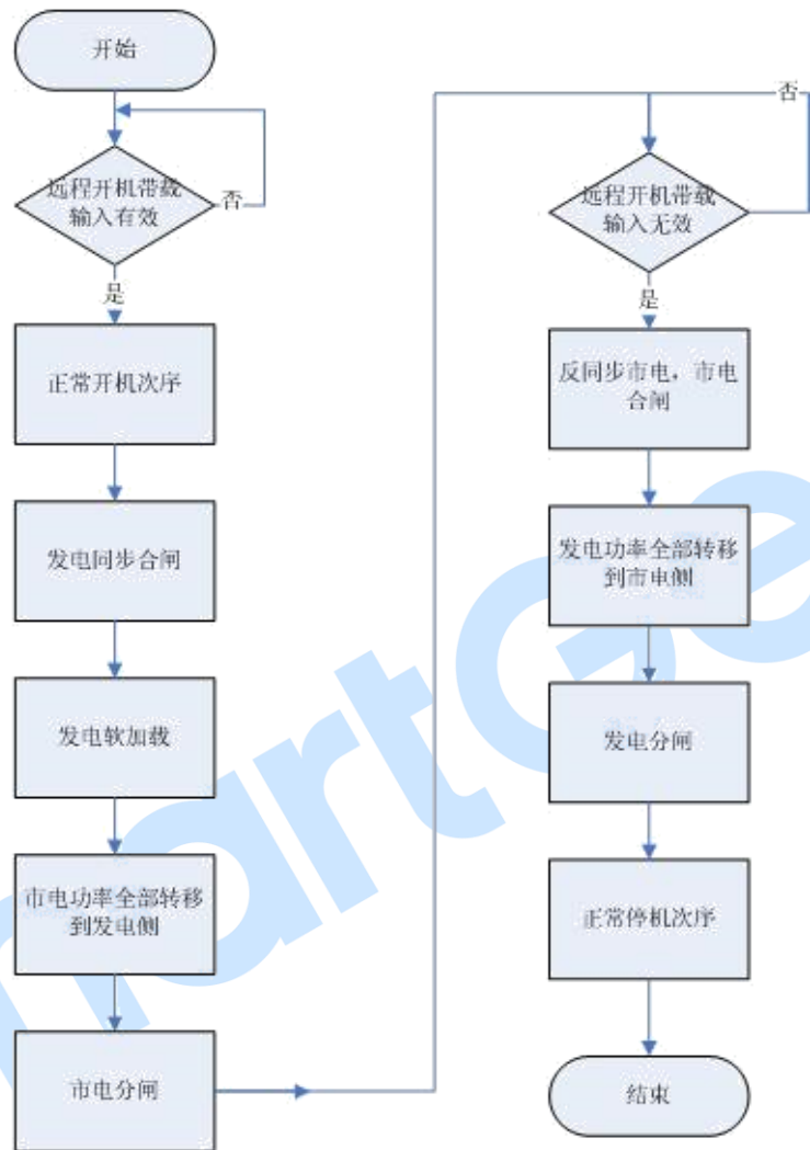
图7 负载接收模式
