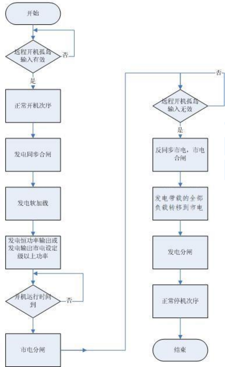
图9 孤岛输出模式
