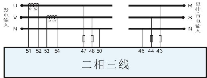
图12 二相三线应用图
