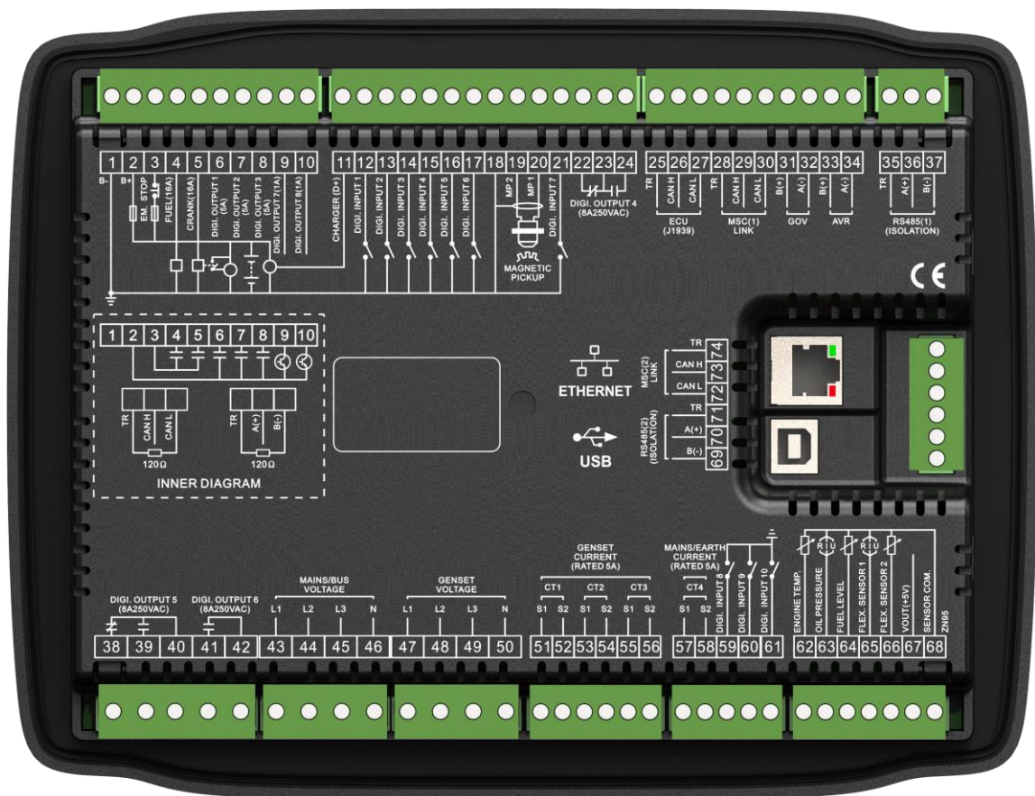
图3 HGM9520N 控制器背面板
