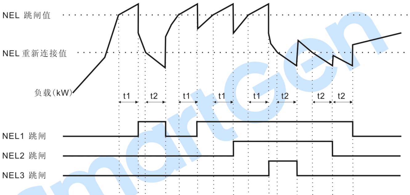
图15 NEL 时序
