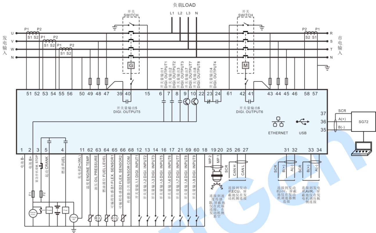
图10 HGM9520N 三相四线典型应用图
