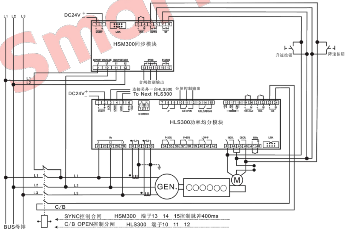
图5 HSM300-HLS300 三相三线典型应用图
