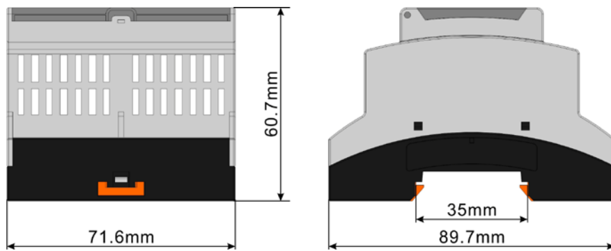
图6 外形尺寸图
