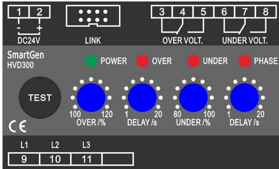
图1 面板图
