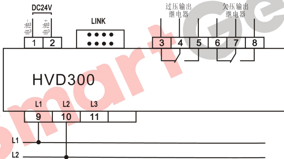
图4 单相两线、两相三线
