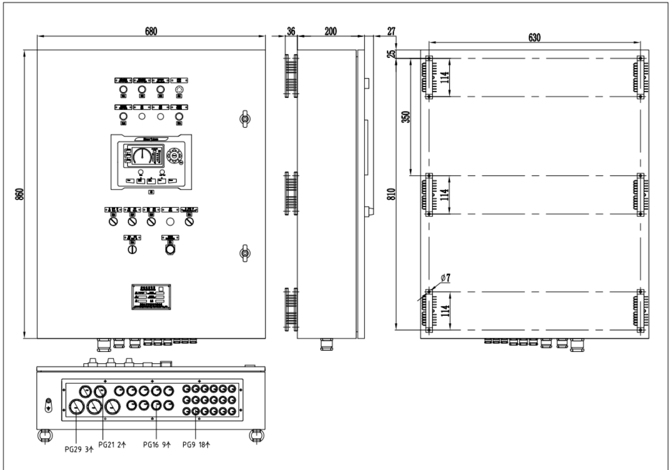
图 2 — 控制箱安装尺寸
