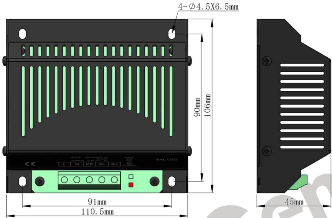
图3 BAC2405CF 安装尺寸图
