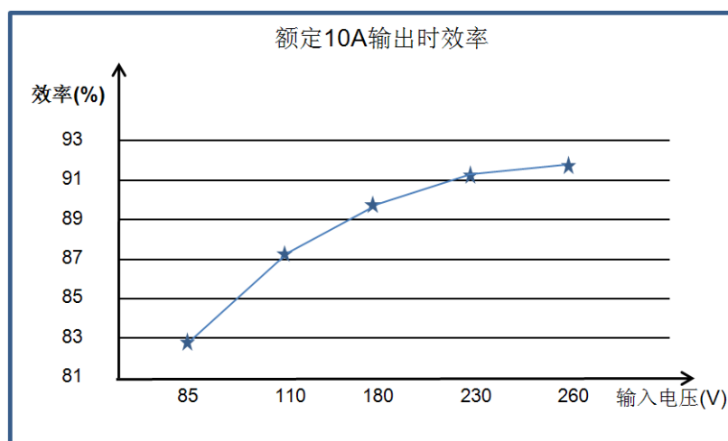
图2 效率曲线
