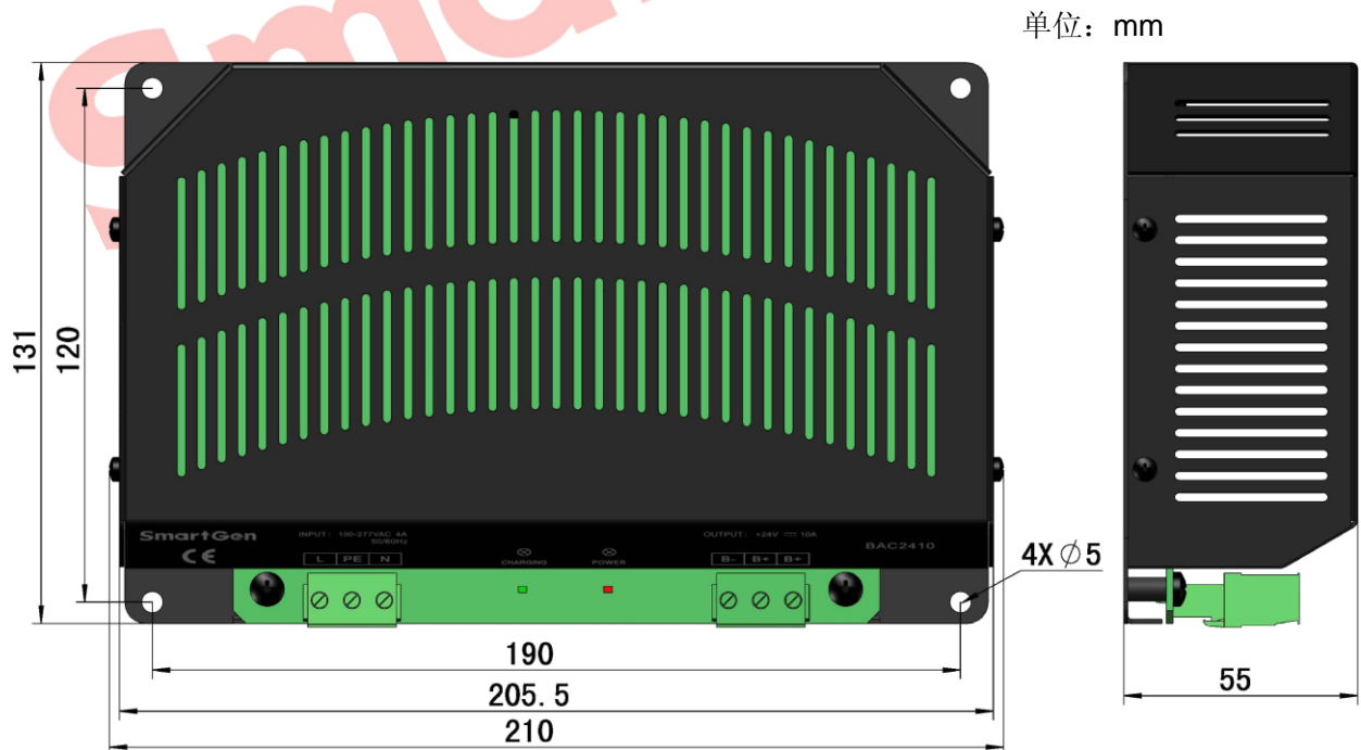
图4 BAC2410 安装尺寸图
