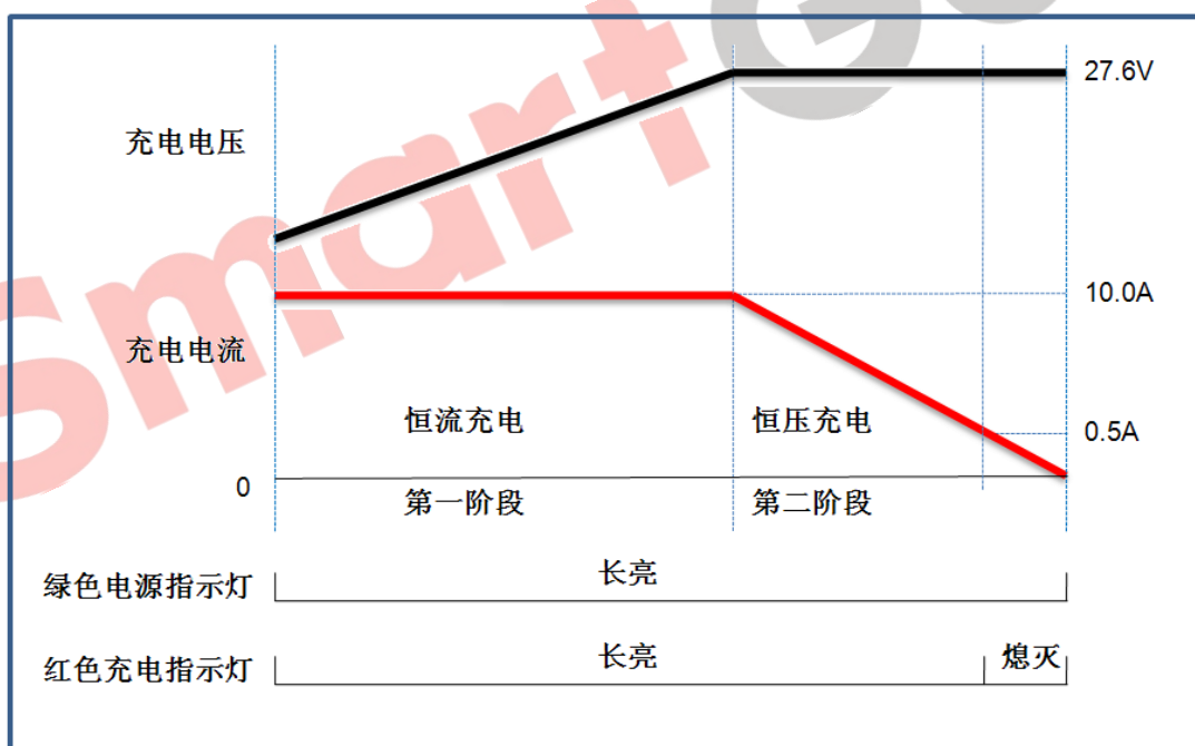
图1 二段式充电曲线图
