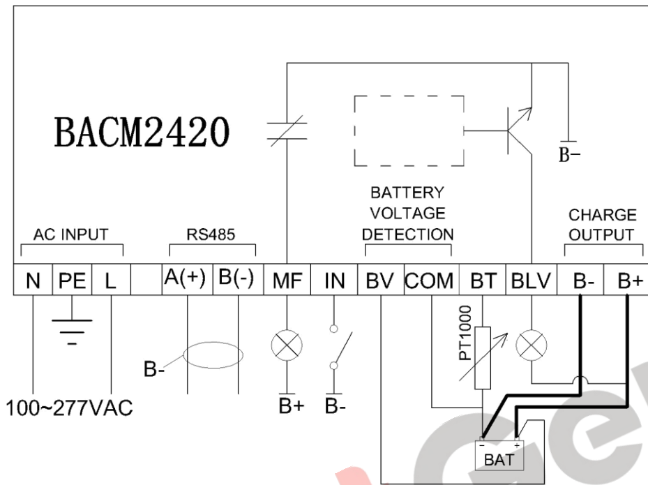
图5 接线图
