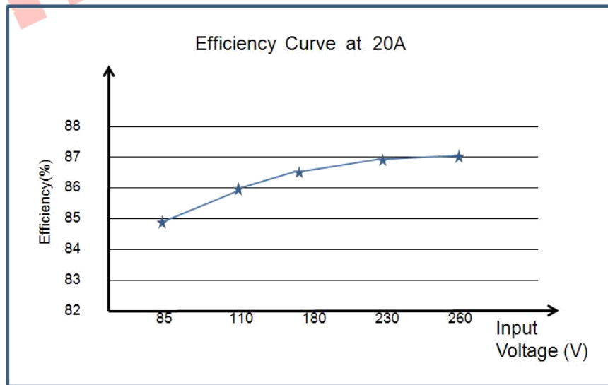
图3 效率曲线
