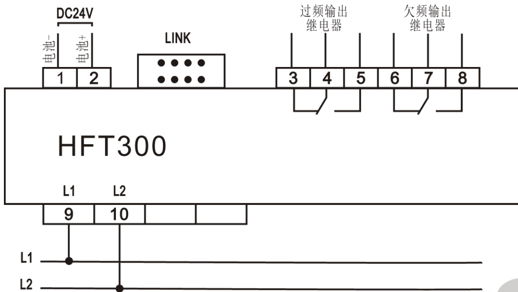
图3 典型应用图
