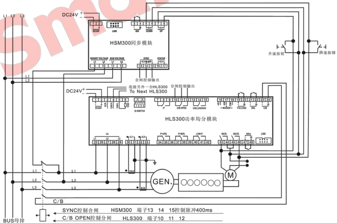
图4 HSM300-HLS300 三相三线典型应用图
