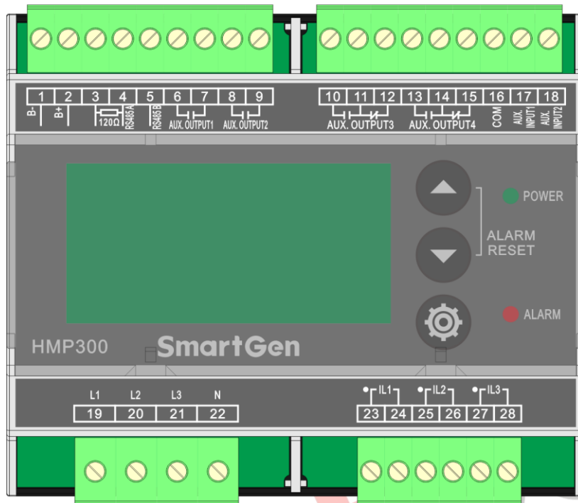
图1 模块面板图
