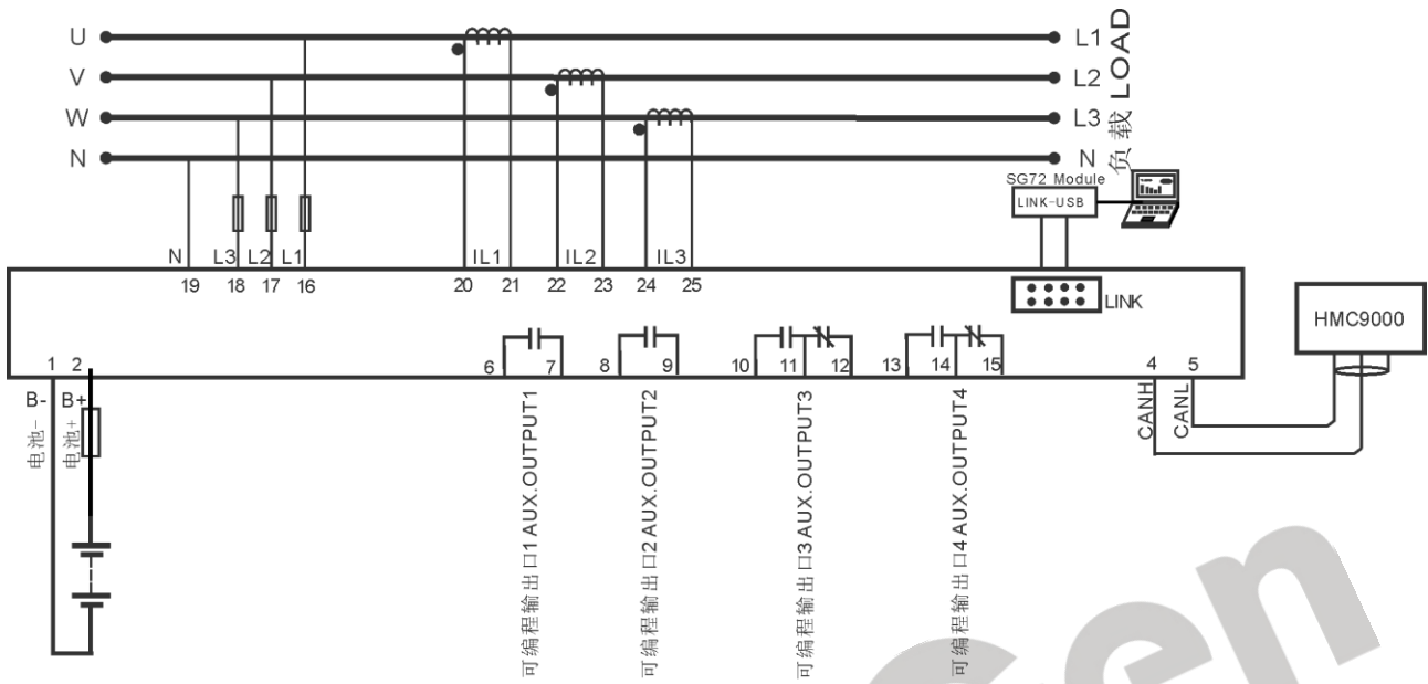
图2 HMP300 典型应用图
