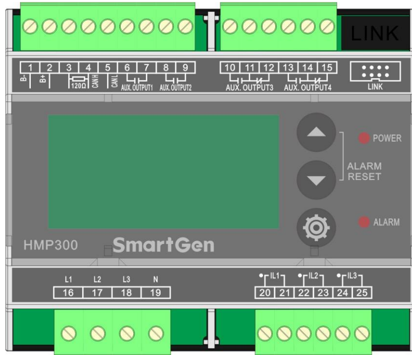
图1 模块面板图
