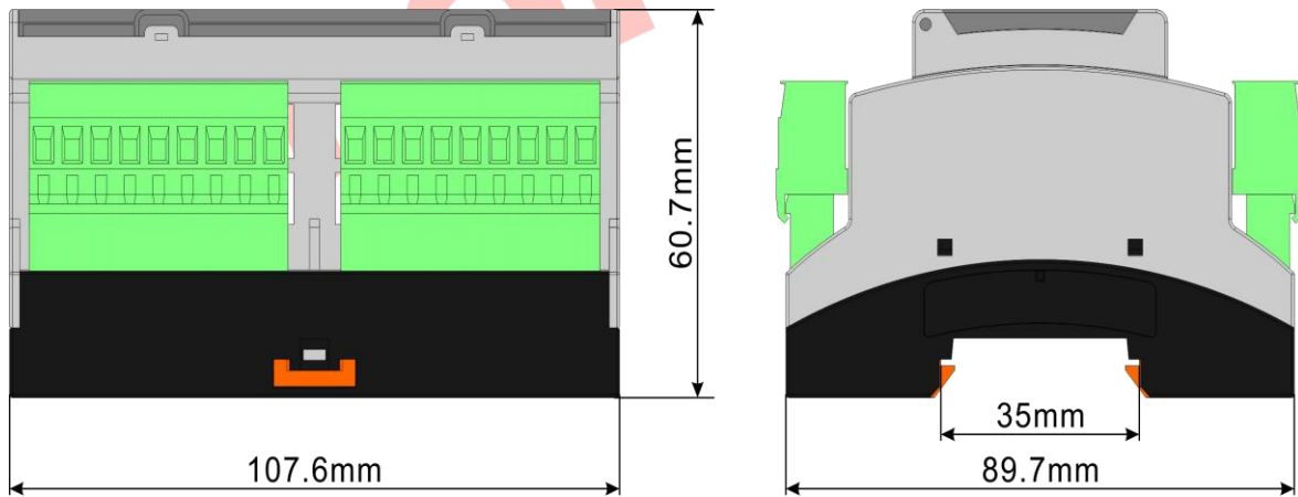
图3 外形及开孔尺寸
