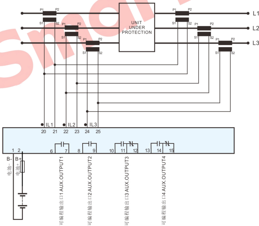
图3 差动保护应用图
