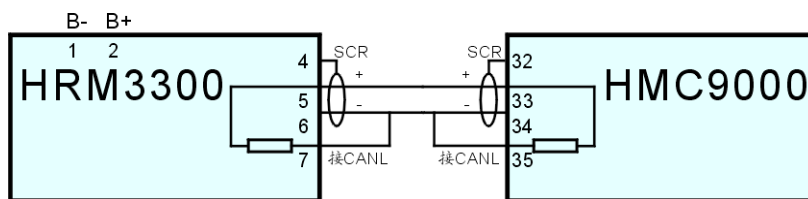
HRM3300 典型接线图
