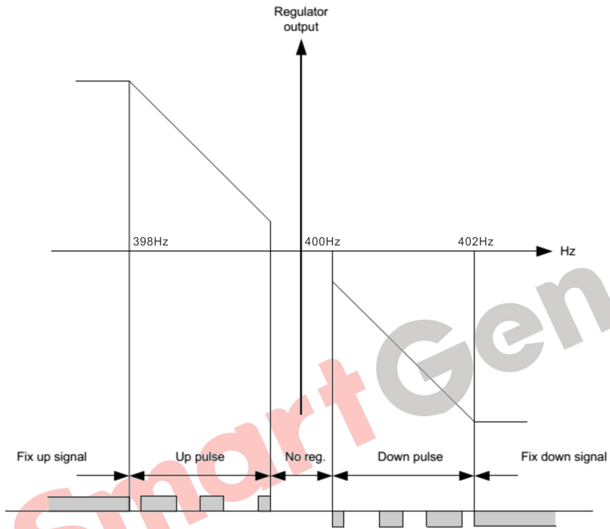
图3 升/降速继电器工作原理图
