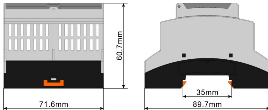
图5 外形尺寸图
