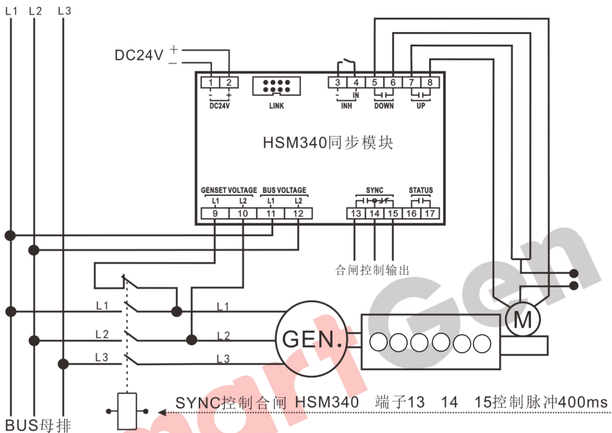
图4 HSM340 三相三线典型应用图
