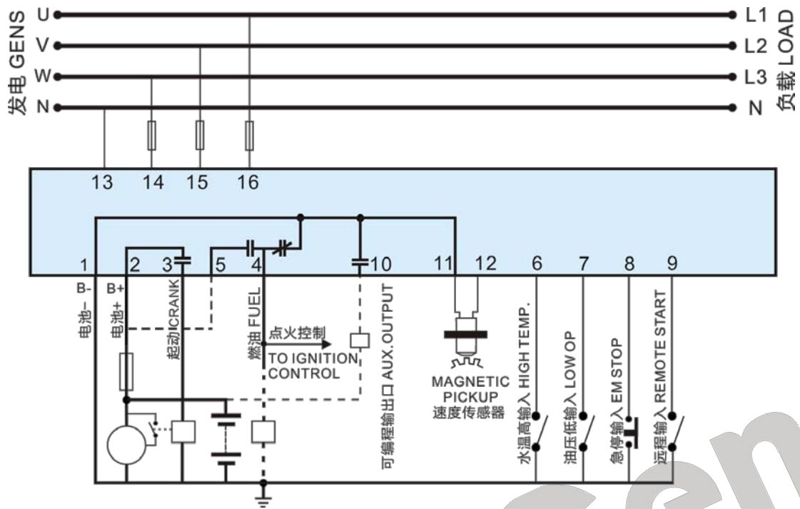
图4 控制器与发电机组连接图
