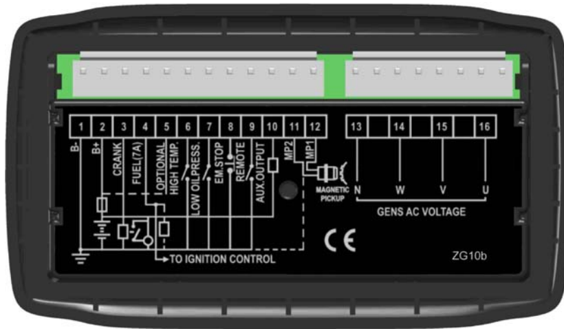
图2 控制器背面板图
