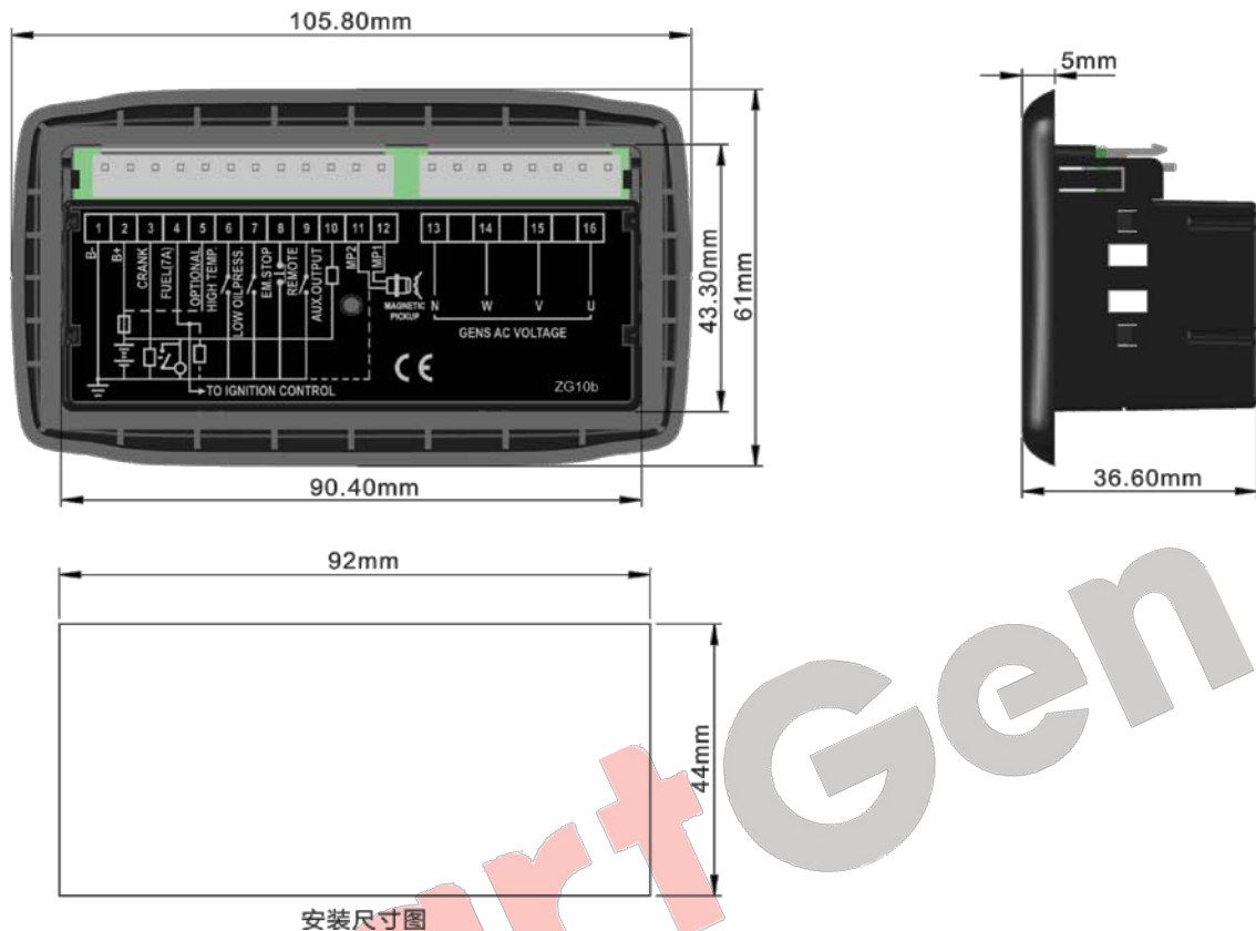
图3 外形尺寸
