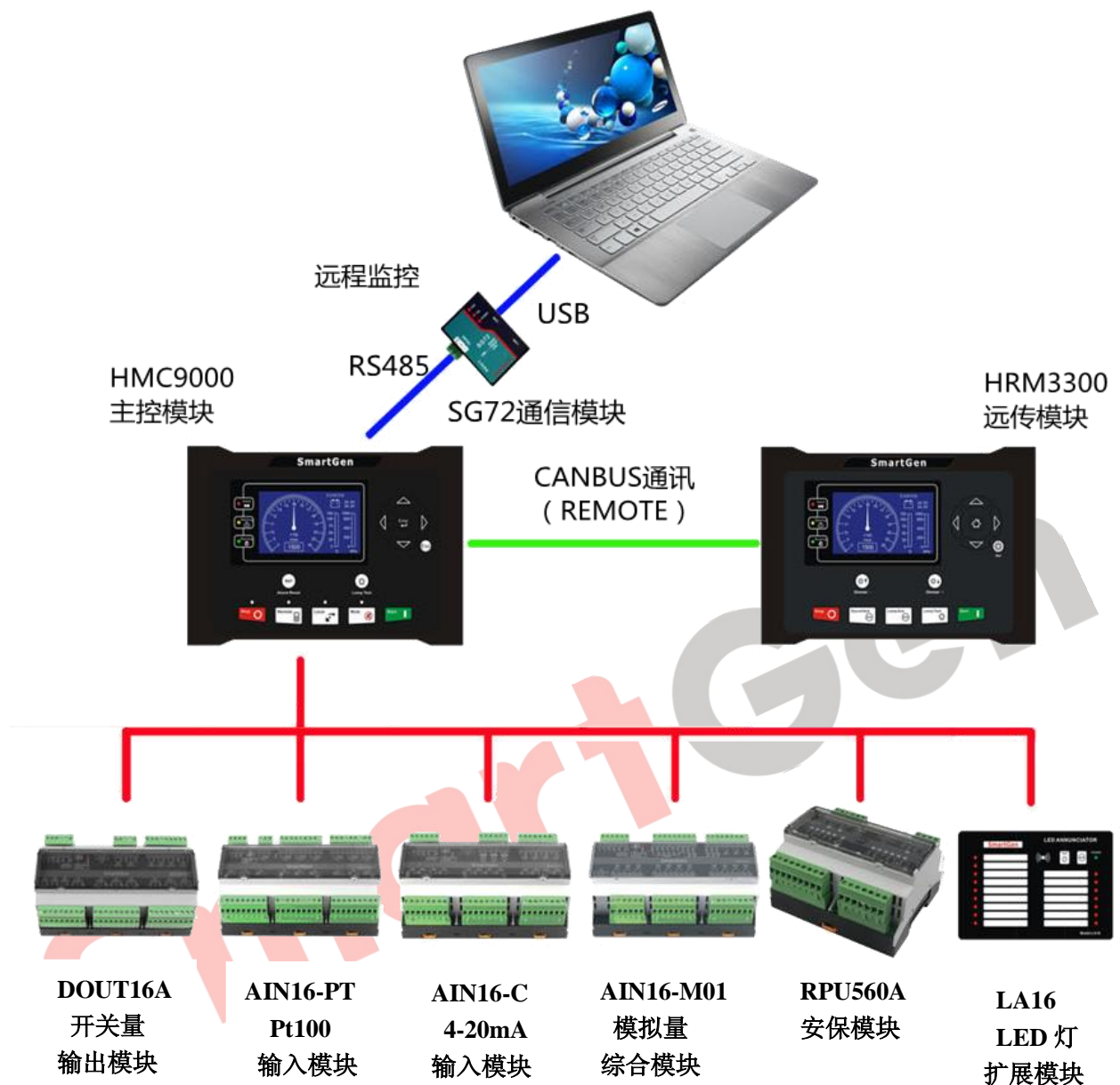
图 3 系统接线图
