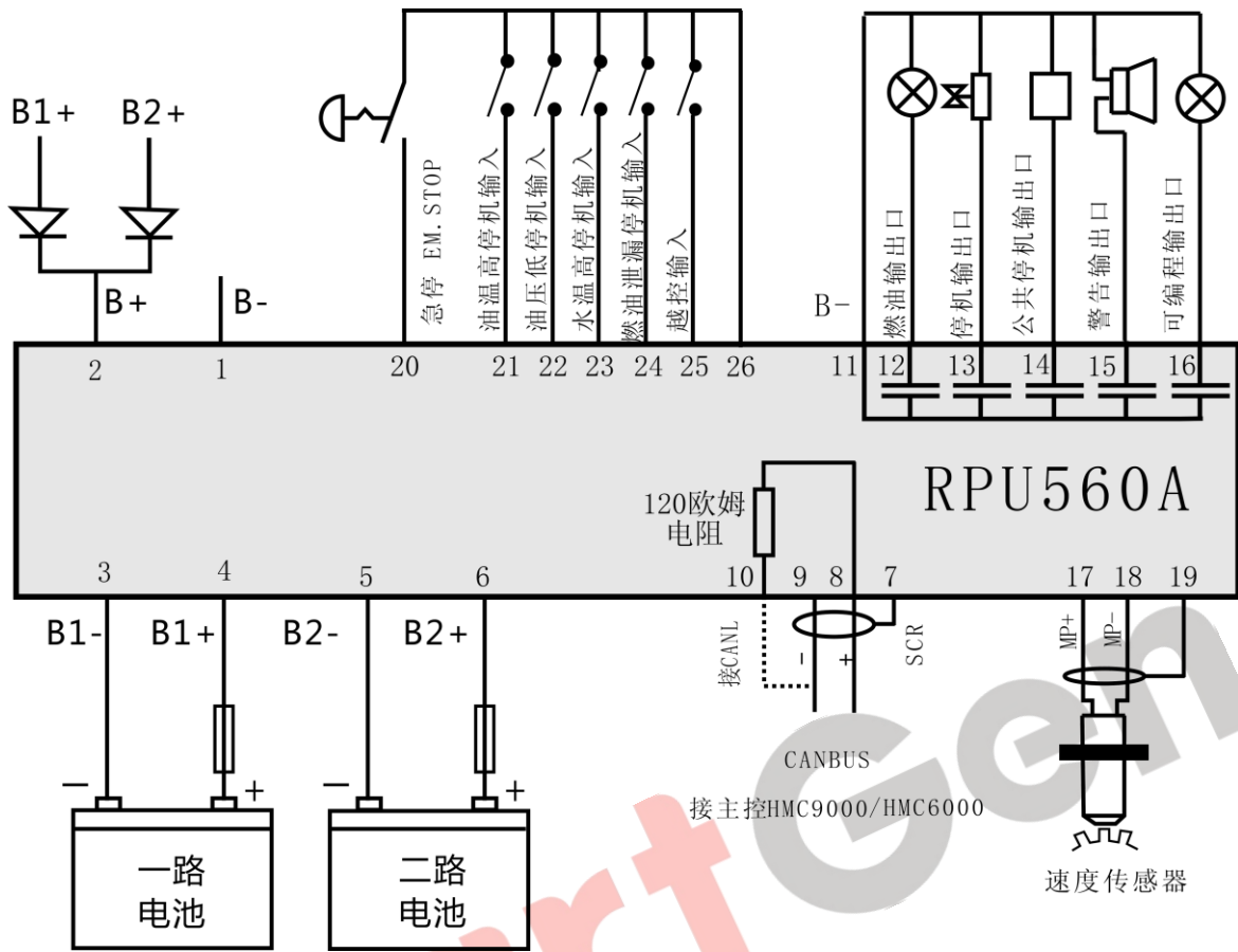
图 4 典型应用图
