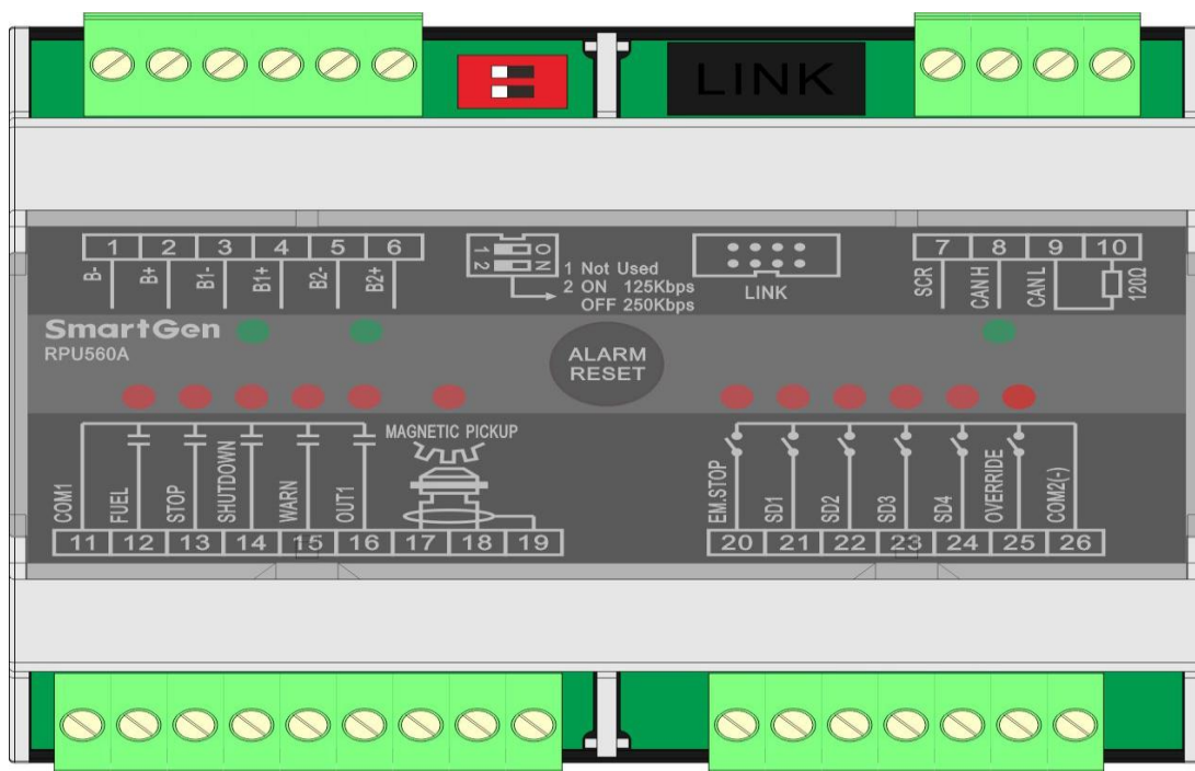
图 2 接线端子描述图
