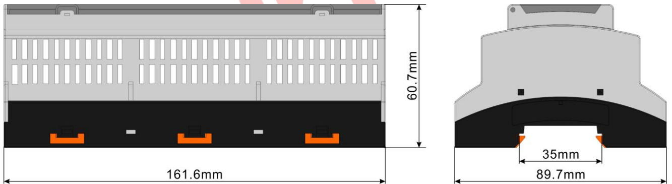
图3 外形尺寸
