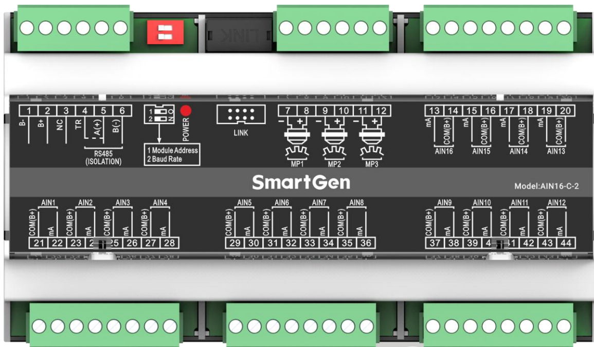
图1 AIN16-C-2 面板图
