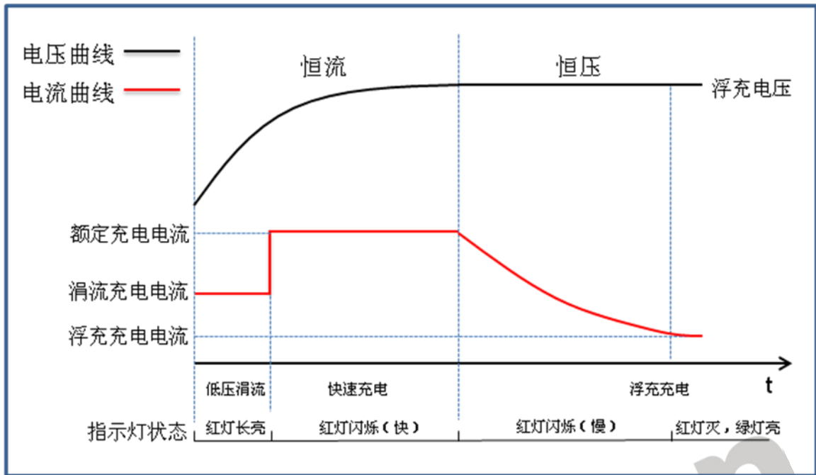
二段式充电曲线图
