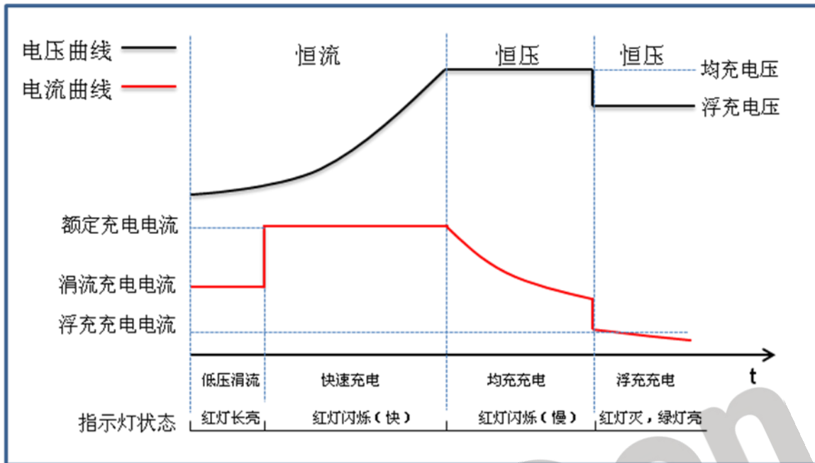
三段式充电曲线图
