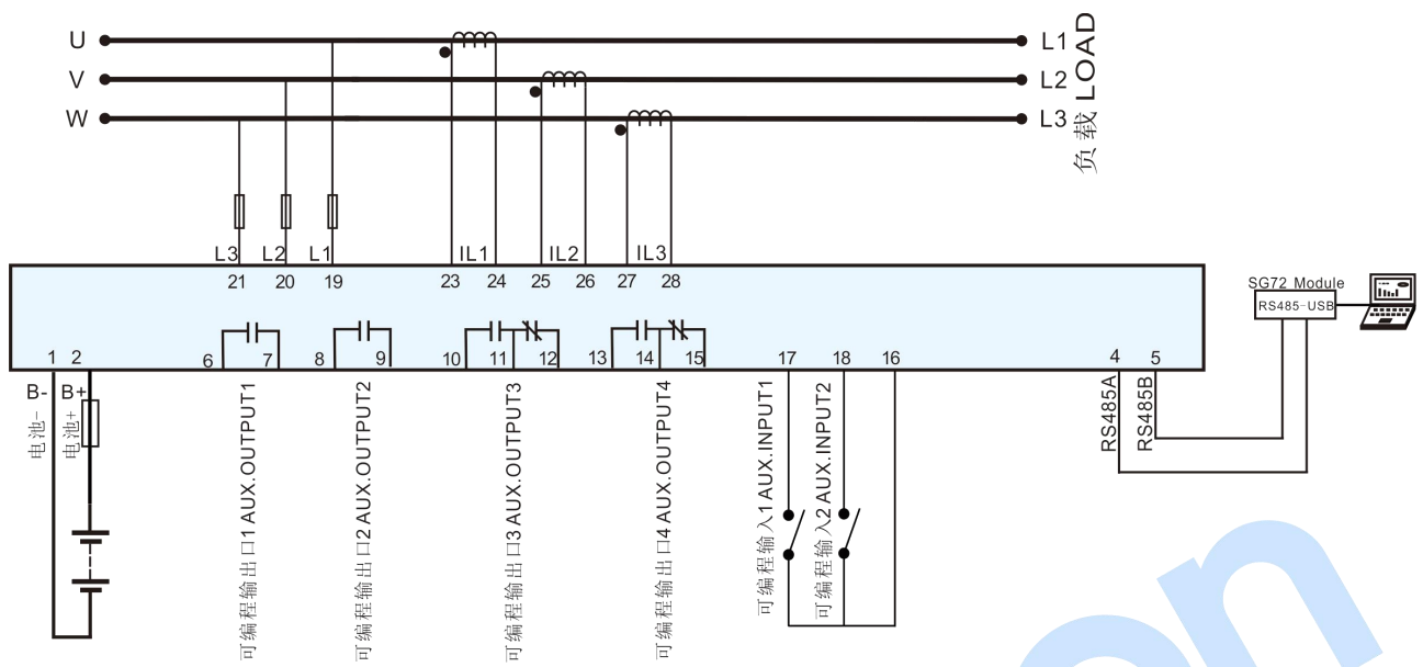
图 3 HMP300 典型应用图
