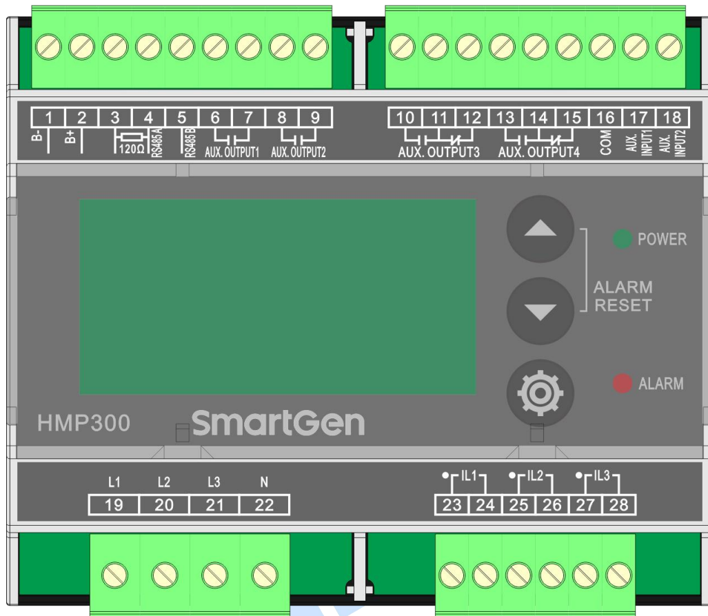
图 1 模块面板图
