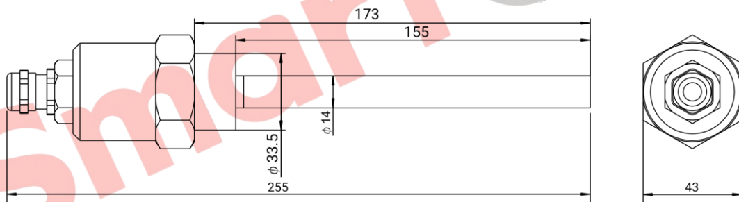
图2 HTL04A 外形及安装尺寸
