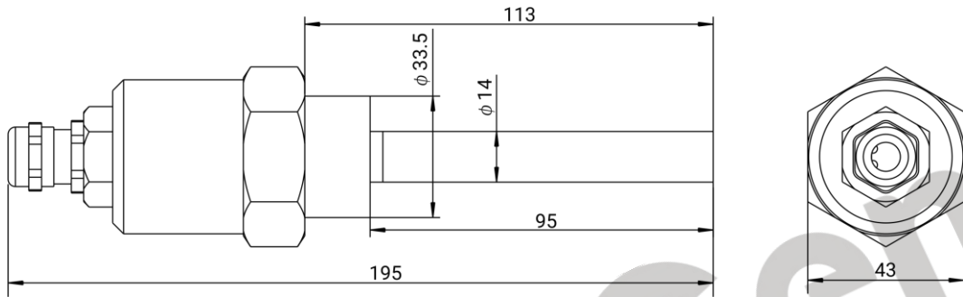
图1 HTL02A 外形及安装尺寸
