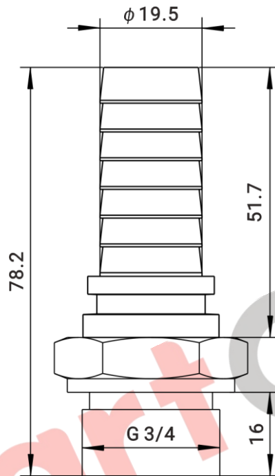
Fig. 8 Pagoda Header Size
