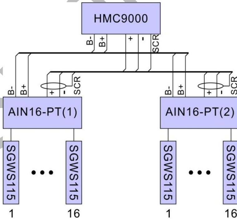
两个 AIN16-PT 和 HMC9000 电气连接图
