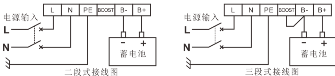
图5 BAC06NB 接线图
