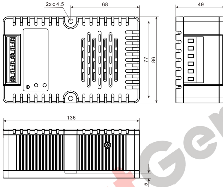
图6 安装尺寸图
