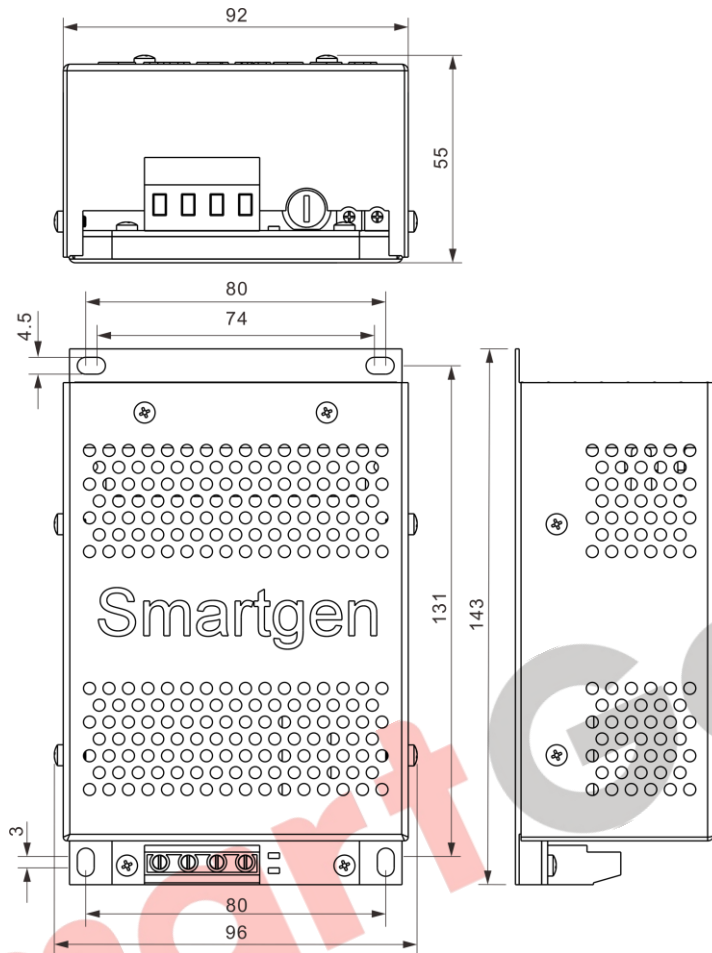
图3 外形及安装尺寸
