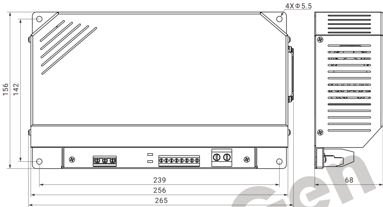
图6 BACM2420A 安装尺寸图
