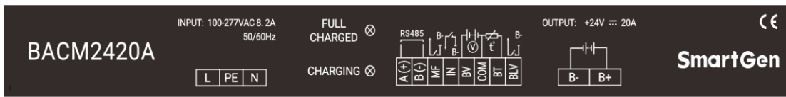
图4 BACM2420A 面板图
