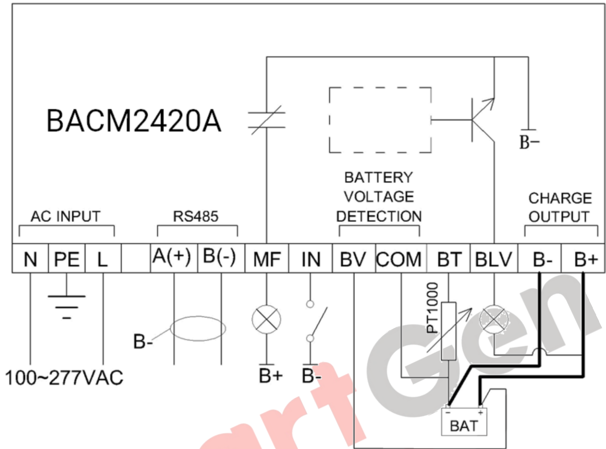
图5 接线图
