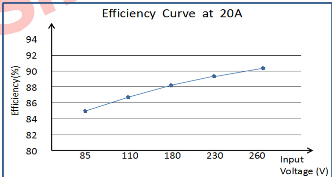
图3 效率曲线
