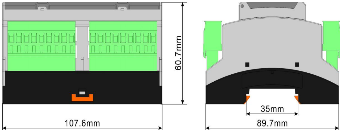
图 3 安装尺寸图
